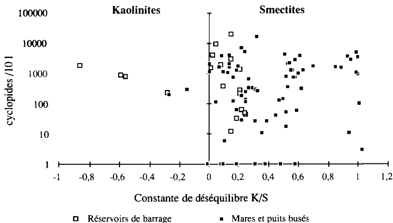
Fig. 2. Relation entre la densité de Cyclopidés et la valeur de la constante de déséquilibre Kaolinites/Smectites. * Fig. 2. Relationship between Cyclopid density and the value of the ration kaolinites.
