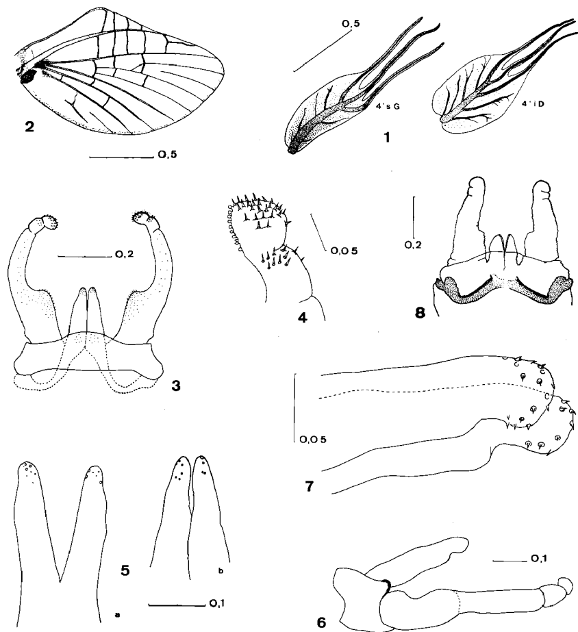
Fig. 1 à 8 : Choroterpes (Euthraulus) lindrothi Peters. Echelle en mm.
