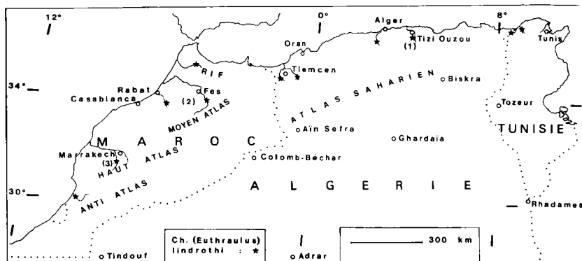
Fig. 9 : répartition de Choroterpes (Euthraulus) lindrothi Peters en Afrique du Nord (références citées d'Ouest). Matériel larvaire seulement, sauf la citation du Rif (élevage) : une seule mention par cours d'eau principal.
